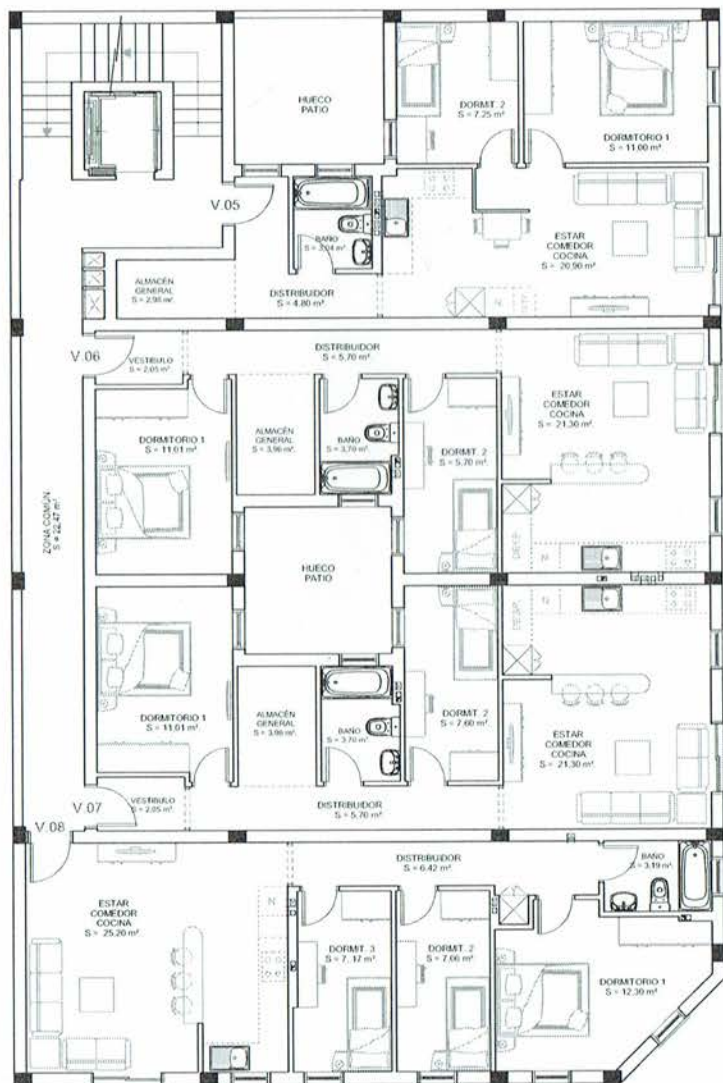
PLANTA PRIMERA. DISTRIBUCIÓN Y SUPERFICIES
