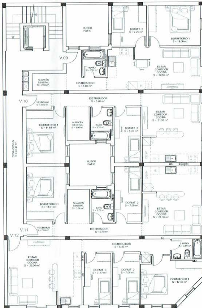
PLANTA SEGUNDA. DISTRIBUCIÓN Y SUPERFICIES
